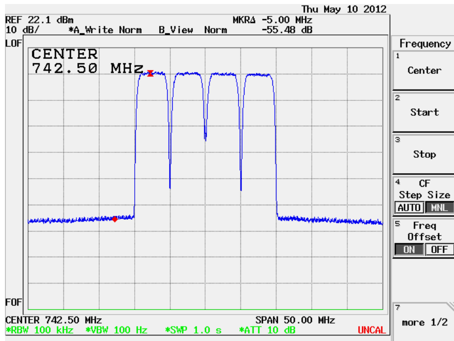
< WCDMA 4FA >
