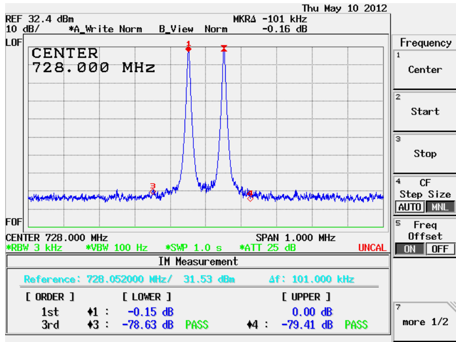
< IMD @ 728MHz >
